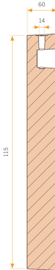
■ Sección transversal
